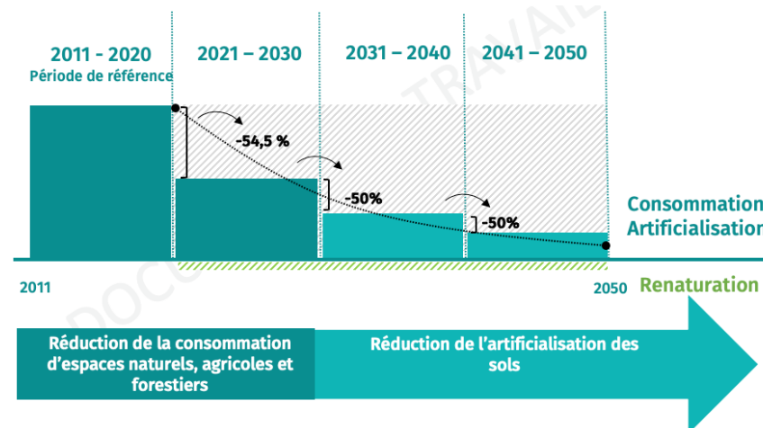
Illustration 2 : Trajectoire de réduction de la consommation d'espaces puis de l'artificialisation
