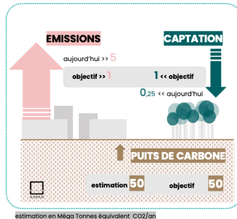
Illustration 4 : Stratégie Nationale Bas Carbone théorique traduite en flux de carbone à l'échelle du Pôle métropolitain Nantes Saint-Nazaire 6
