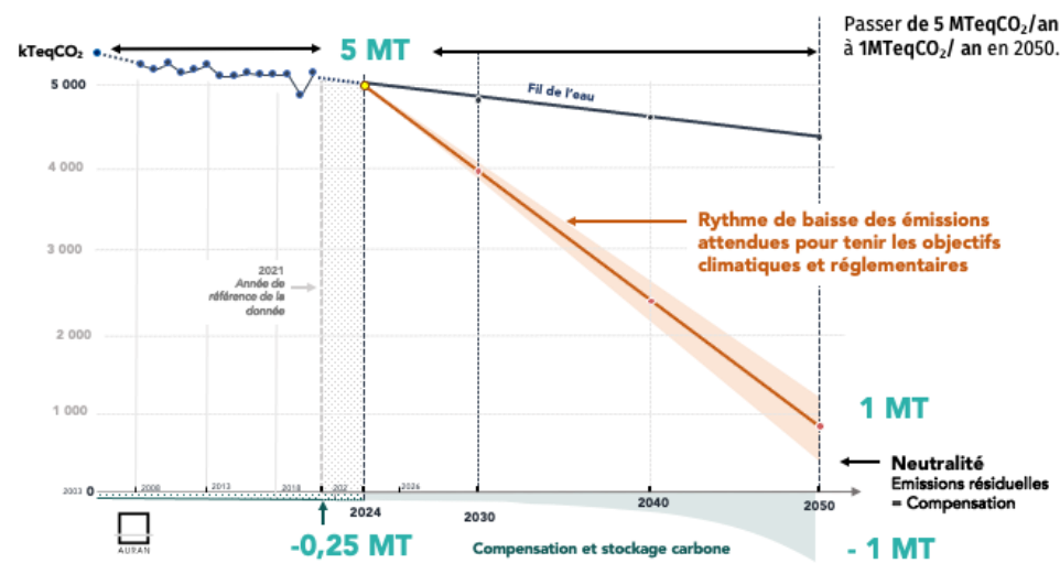
Illustration 3 : Trajectoire théorique de la Stratégie Nationale Bas Carbone traduite à l'échelle du territoire Nantes Saint-Nazaire 3
